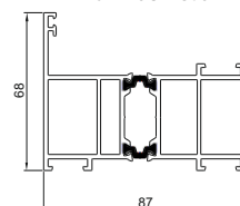
Profil naświetla
