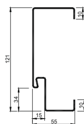
Ościeznica stalowa S15/54
