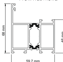
Profil naświetla
