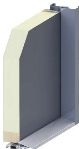
75 PASSIVE (zewewnętrzne)
