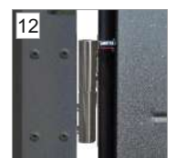
Trzy zawiasy 3D z nasadką, regulowane w trzech płaszczyznach
