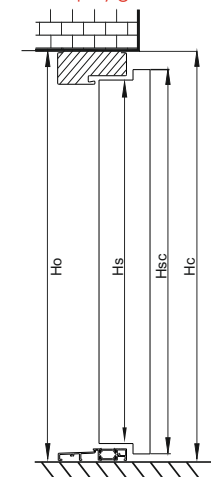
Drzwi cztero przyłgowe 4P
