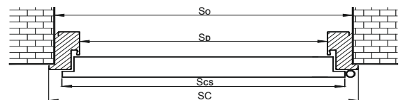
Drzwi trzy przyłgowe 3P
