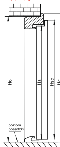
Drzwi trzy przyłgowe 3P
