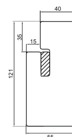
Ościeznica stalowa NT/54, NT/54 AKU
